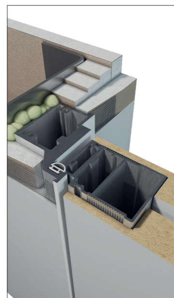
VSTAVANIE DO SADROKARTÓNU - KRÍDLO BEZ RÁFIKA
