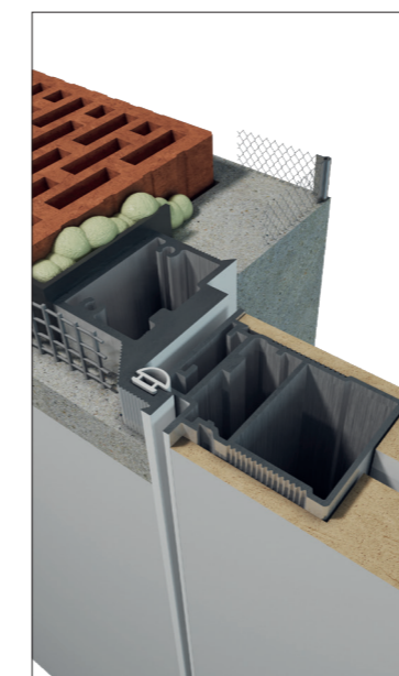
VSTAVANIE DO STENY - KRÍDLO S RÁFIKOM
