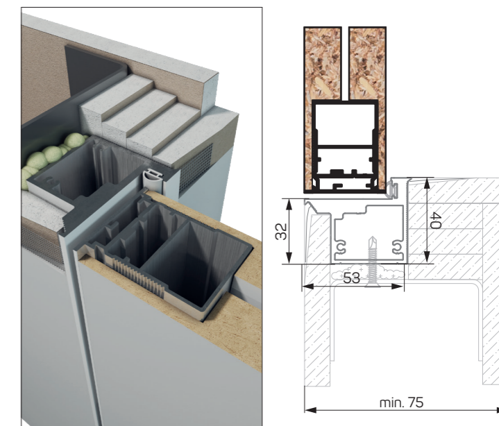
VSTAVANIE DO SADROKARTÓNU - KRÍDLO S RÁFIKOM
