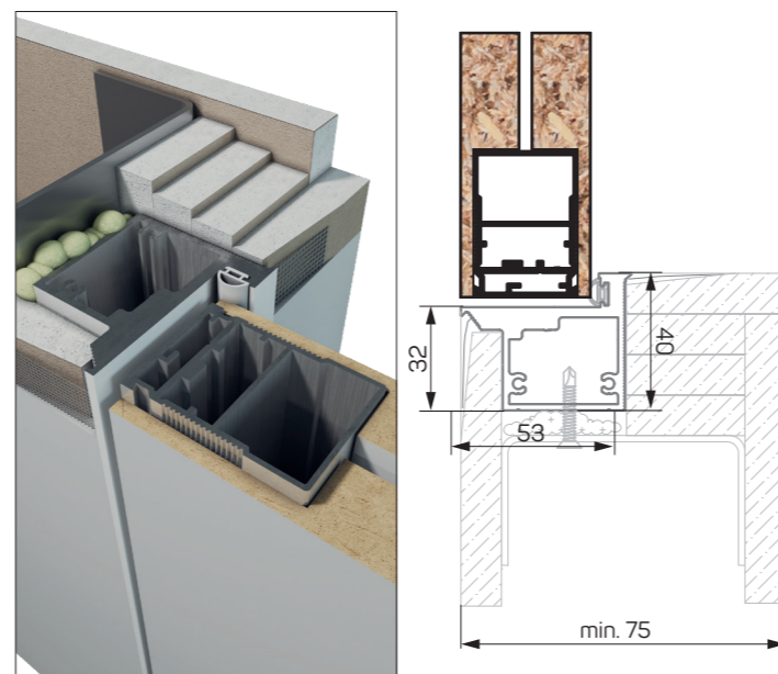
VSTAVANIE DO SADROKARTÓNU - KRÍDLO BEZ RÁFIKA
