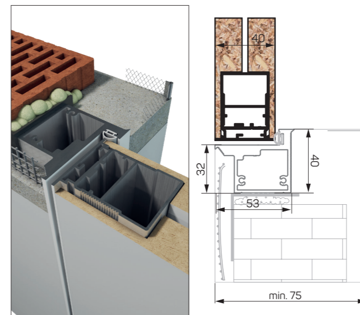
VSTAVANIE DO STENY - KRÍDLO S RÁFIKOM
