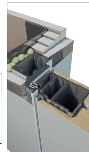
VSTAVANIE DO SADROKARTÓNU - KRÍDLO S RÁFIKOM
