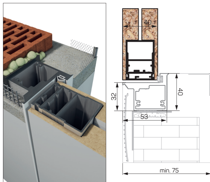
VSTAVANIE DO STENY - KRÍDLO BEZ RÁFIKA
