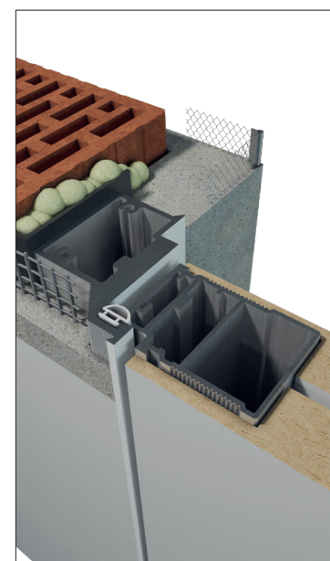
VSTAVANIE DO STENY - KRÍDLO BEZ RÁFIKA
